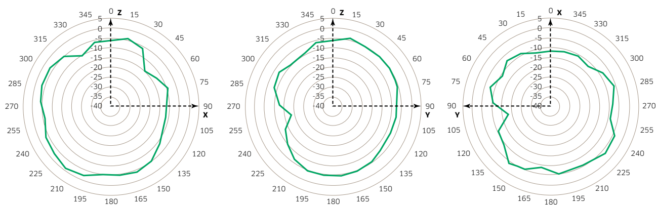
Figura 1. Diagramas de la antena BLE de OmniAccess AP1201
